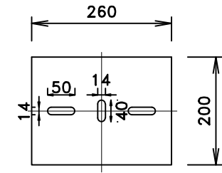
つなぎ板 TGE-26長穴加工 詳細図 S=1:10
