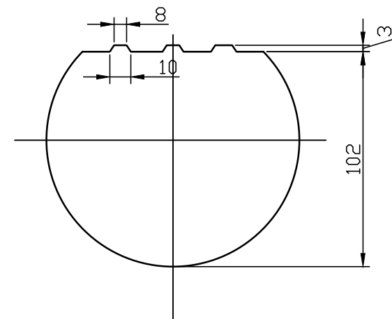
滑り止め形状詳細
