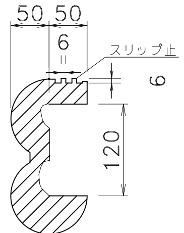
A-A断面 S=1:
